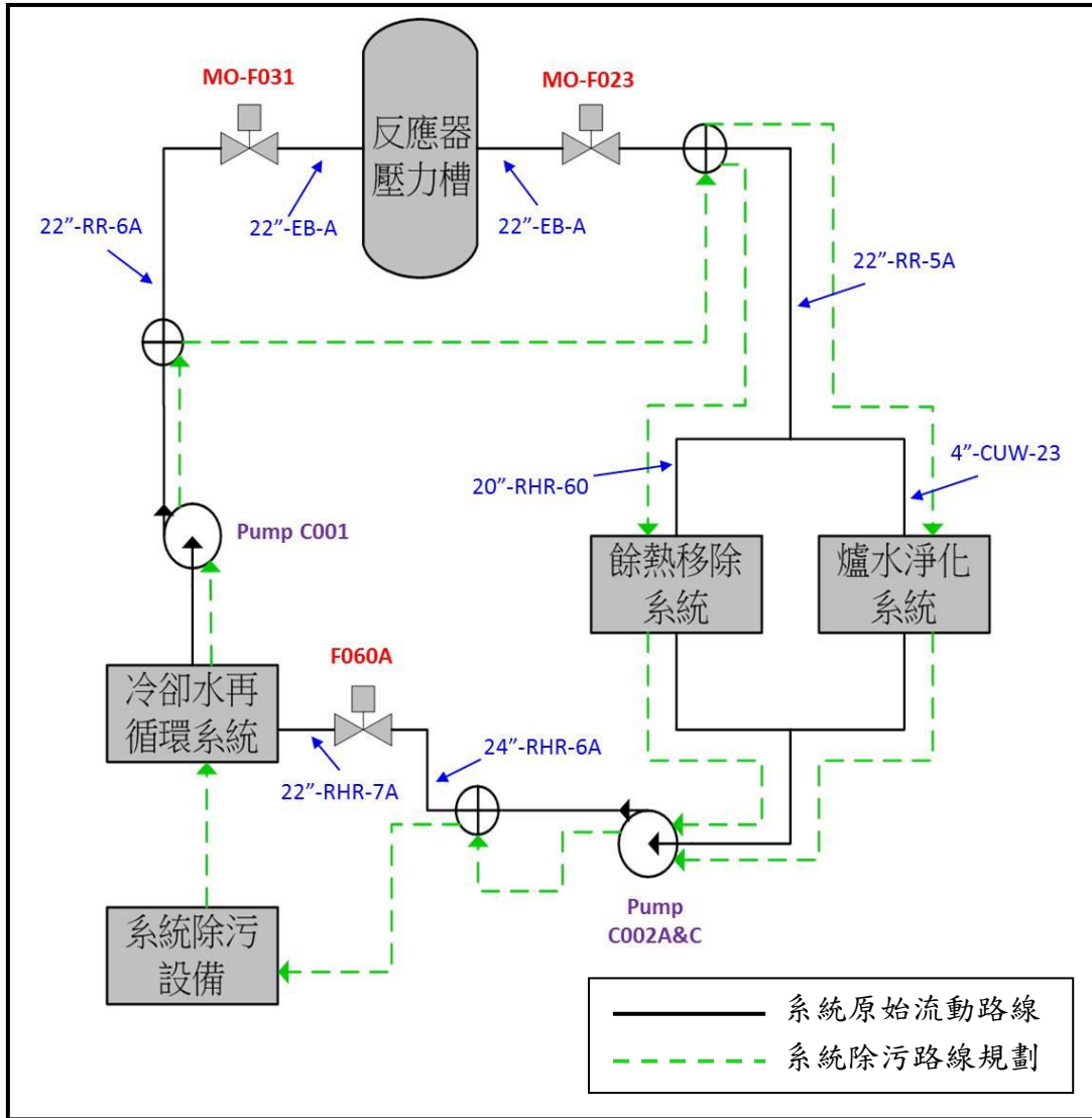
圖 8-1 核一廠系統除污之安裝位置及流程圖
