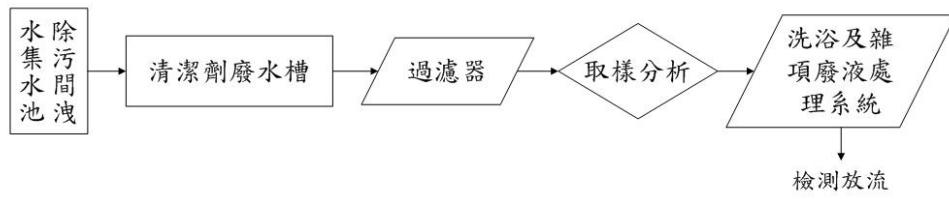
(a)清潔劑廢水系統
