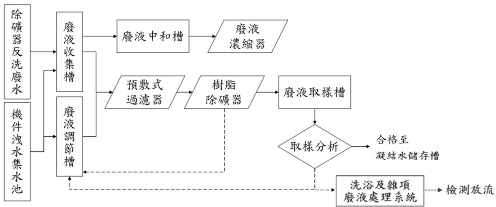
圖 8-6 設備洩水廢液處理系統流程圖
