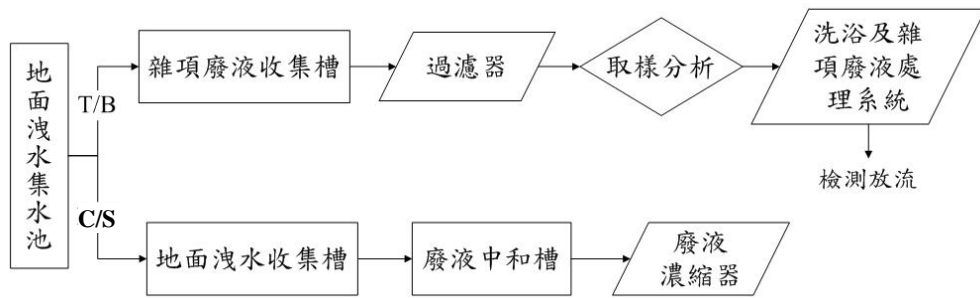
圖 8-7 地面洩水處理系統流程圖
