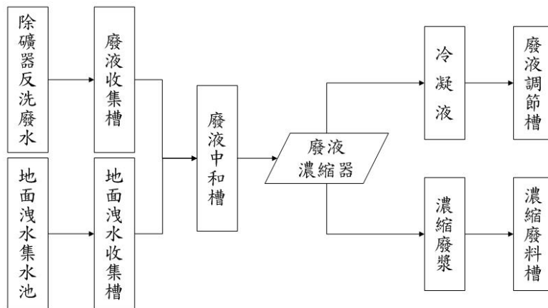
圖 8-8 廢液中和槽與濃縮系統
