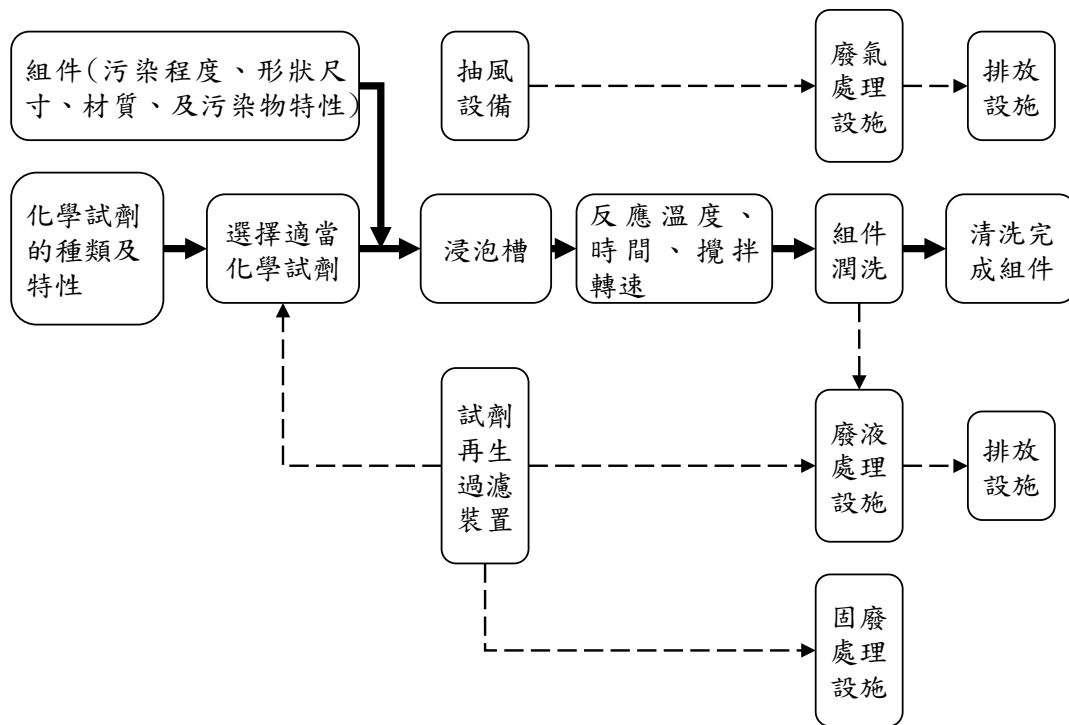
圖 8-2 核一廠金屬類組件之化學除污作業流程示意圖
