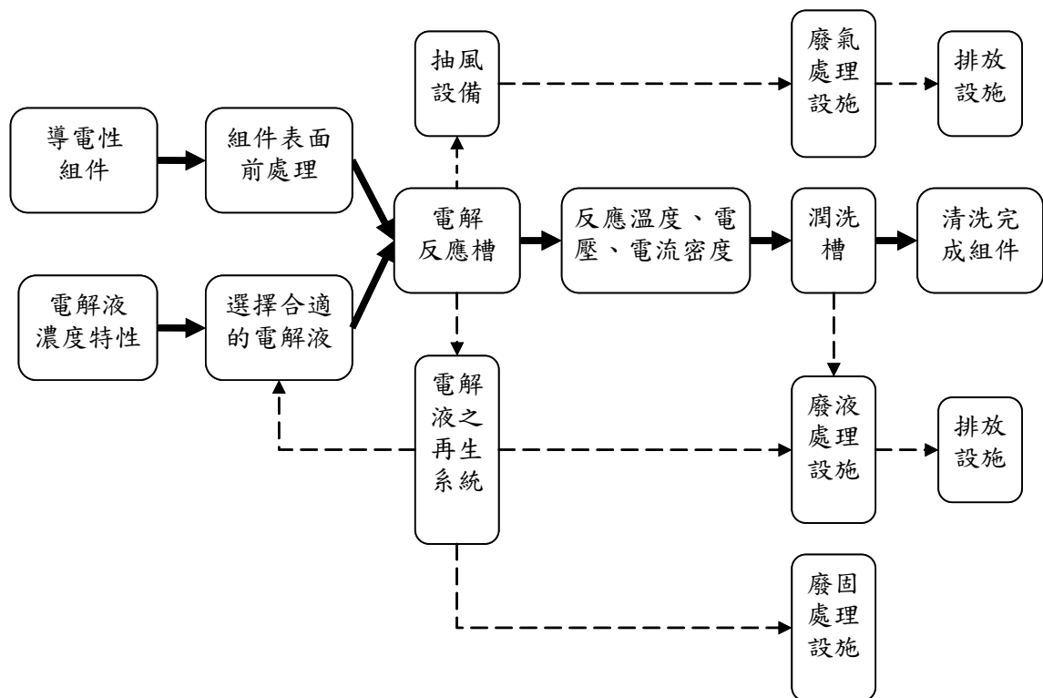
圖 8-3 核一廠金屬類組件之電化學除污作業流程示意圖
