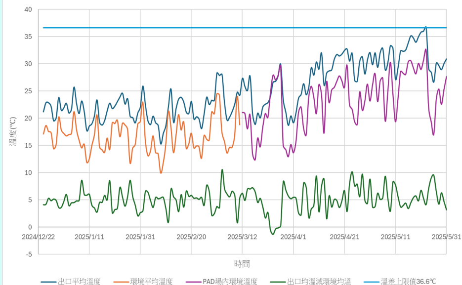
第二組護箱溫度監測
