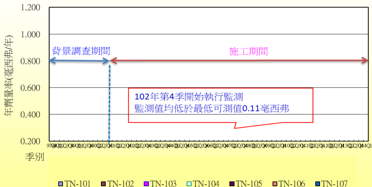
核一廠乾式貯存設施環境輻射監測-貯存場周圍 (中子熱發光劑量計，TLD)
