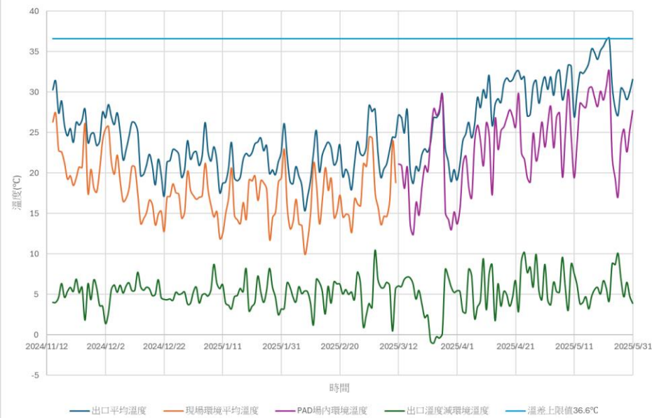
第一組護箱溫度監測
